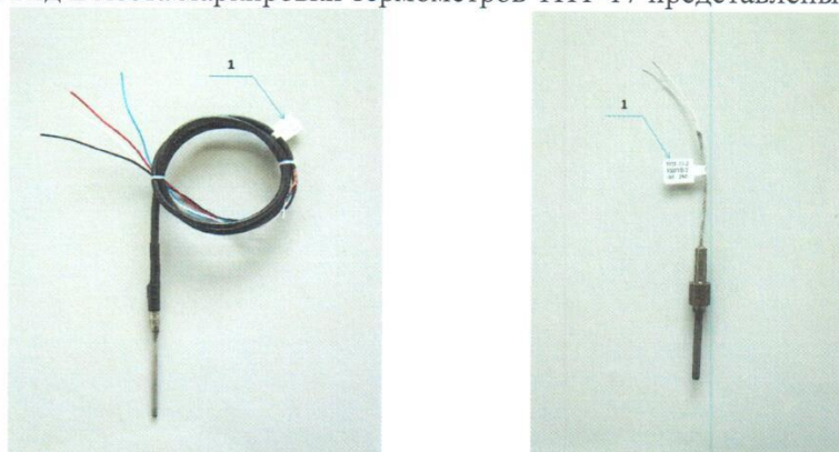
ТПТ-17-1 ТПТ-17-2 Рисунок 2 – Внешний вид термометров ТПТ-17. (1 – место нанесения маркировки)
